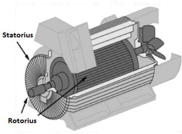
Pav. 4. Generatoriaus pjūvis 2
