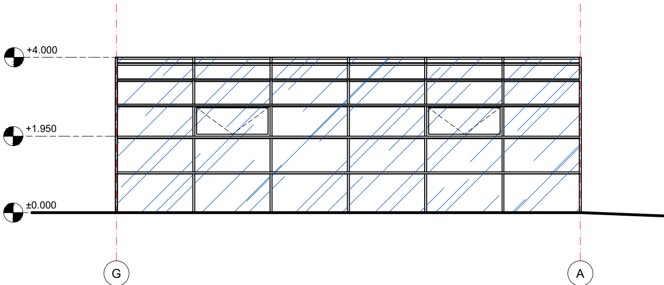
FASADAS G-A M1:100
