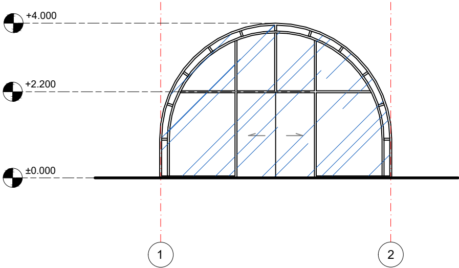
FASADAS 1-2 M1:100
