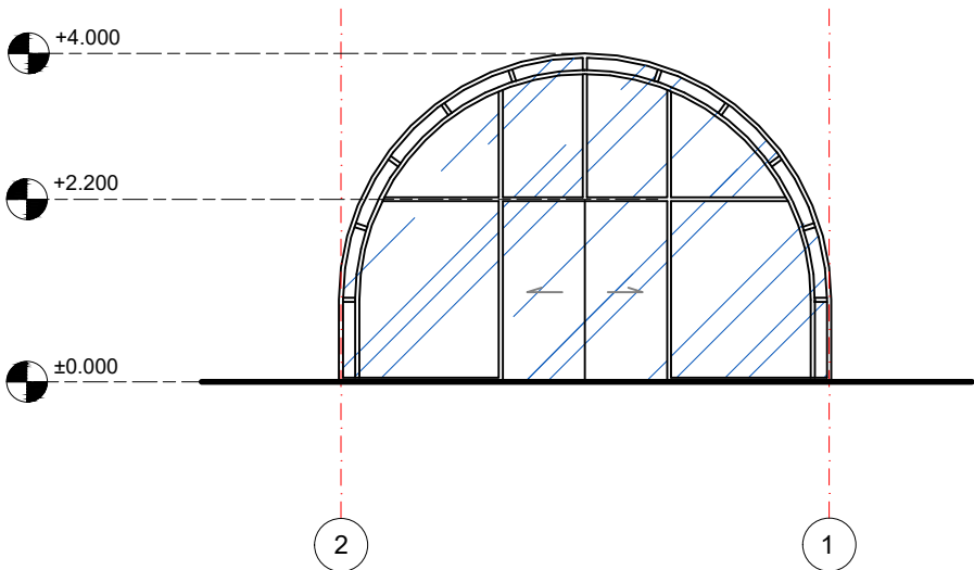
FASADAS 2-1 M1:100
