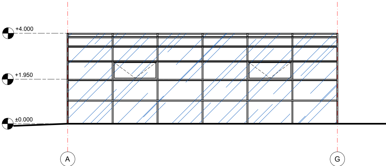
FASADAS A-G M1:100
