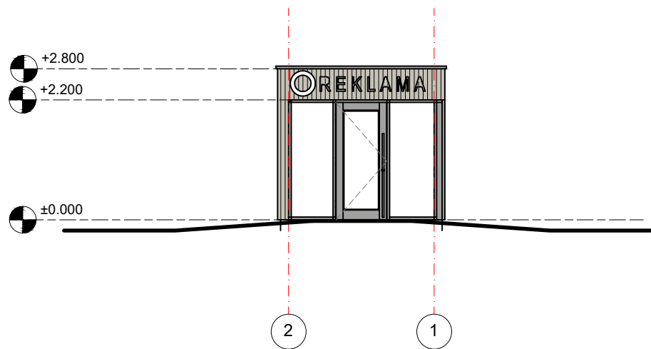
FASADAS 2-1 M1:100
