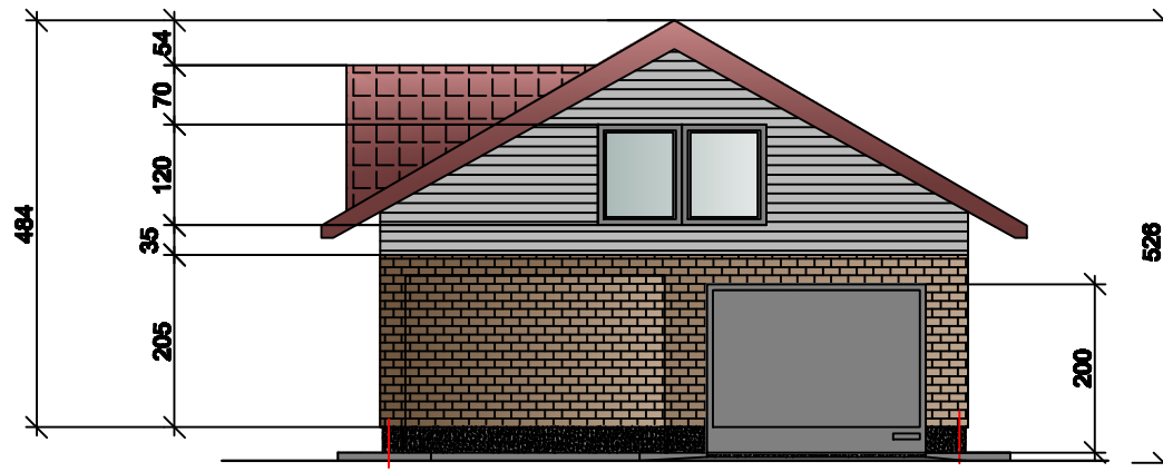
FASADAS 1-3 M 1 : 100
