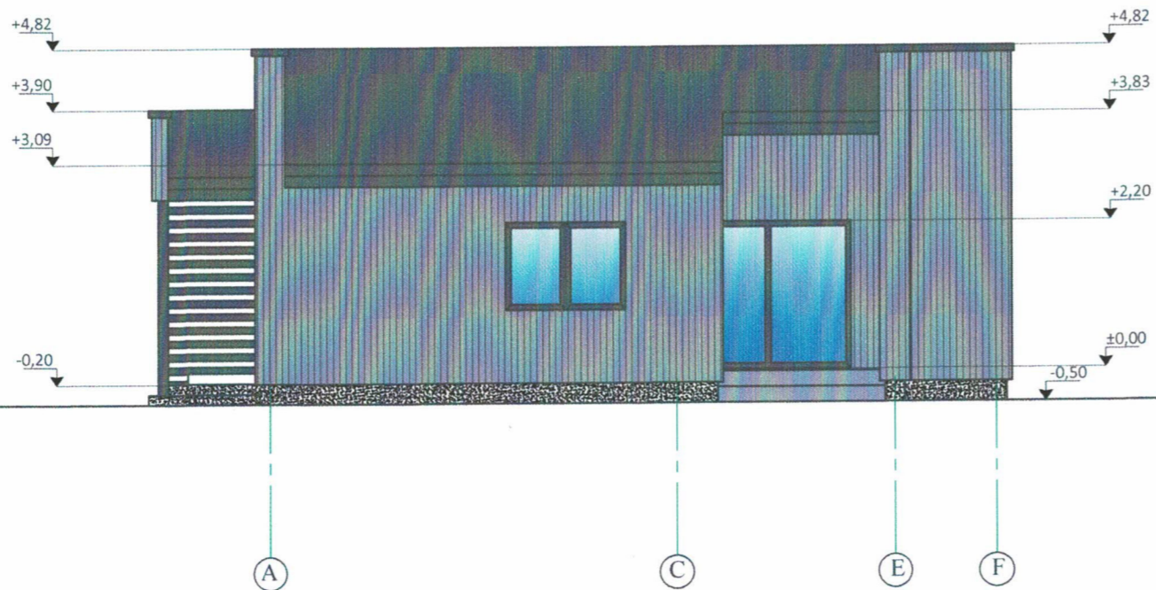
FASADAS A-F M 1:100
