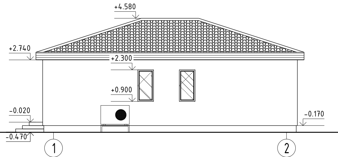
FASADAS 1-2
