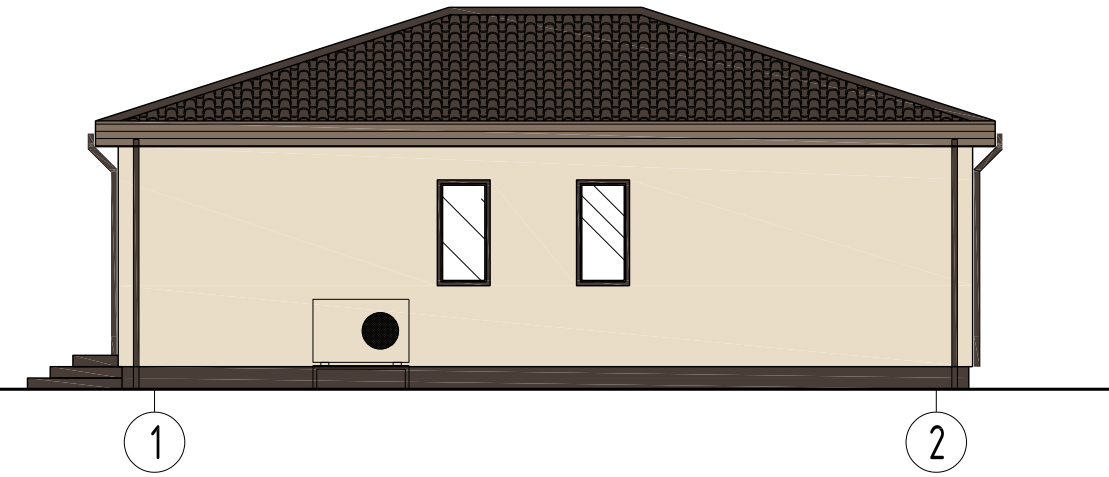
FASADAS 2-1
