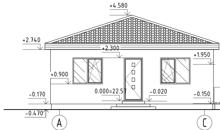
FASADAS A-C
