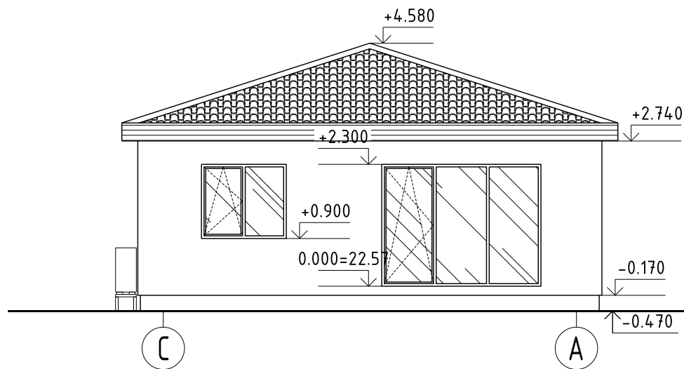
FASADAS C-A
