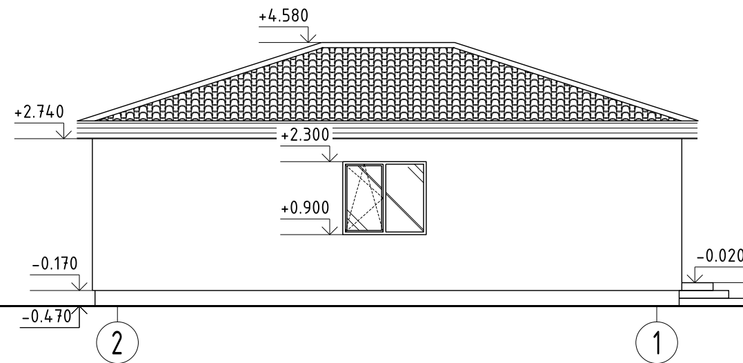
FASADAS 2-1
