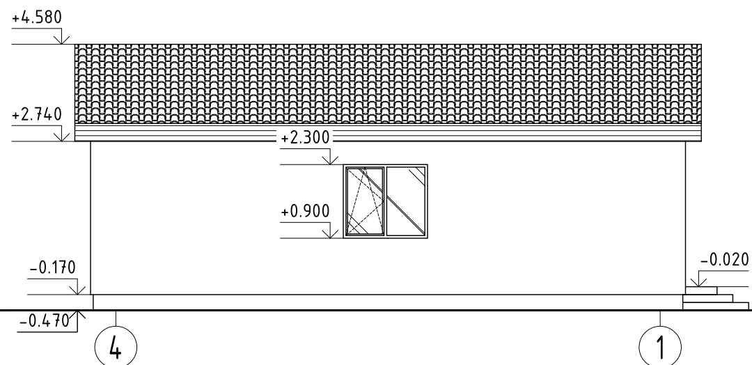
FASADAS 1-4
