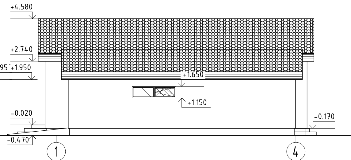
FASADAS 4-1
