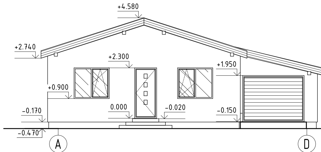
FASADAS D-A
