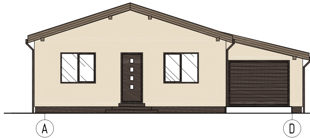
FASADAS A-D
