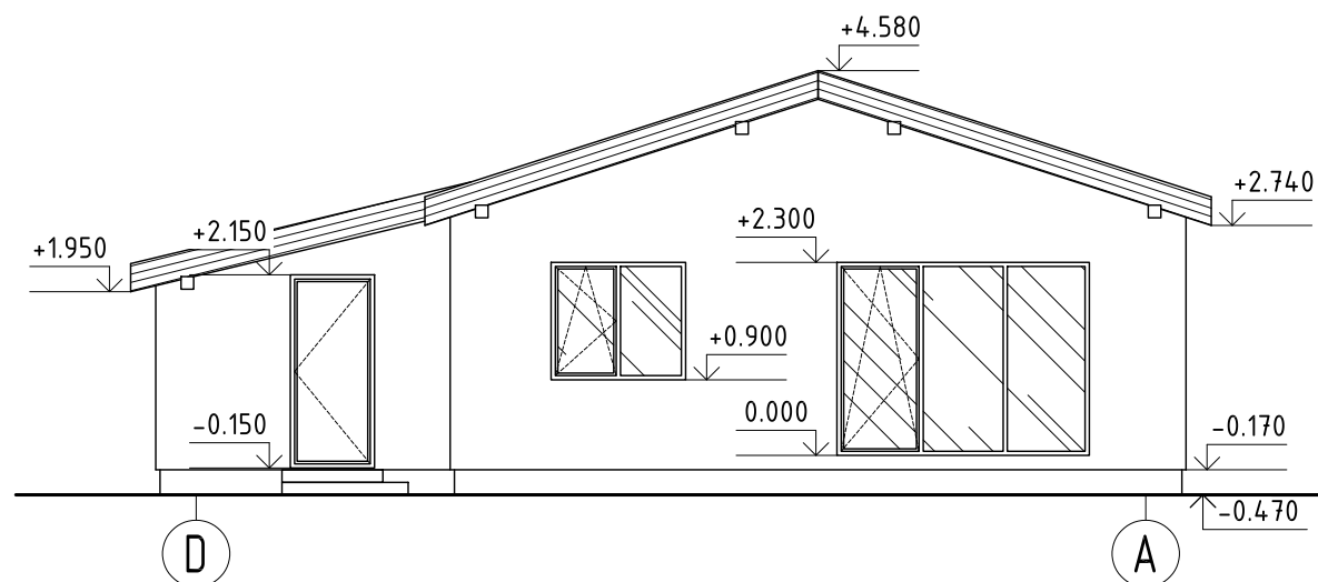
FASADAS A-D
