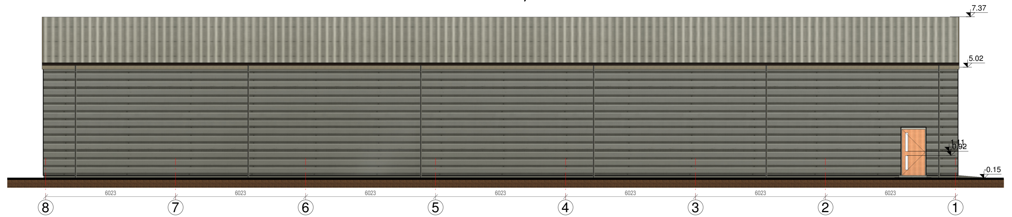
FASADAS 8-1, M 1 : 100
