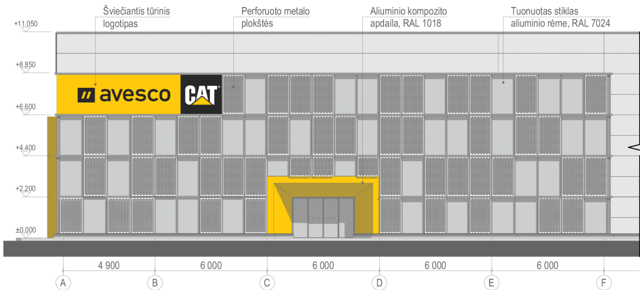
PIETINIS FASADAS
