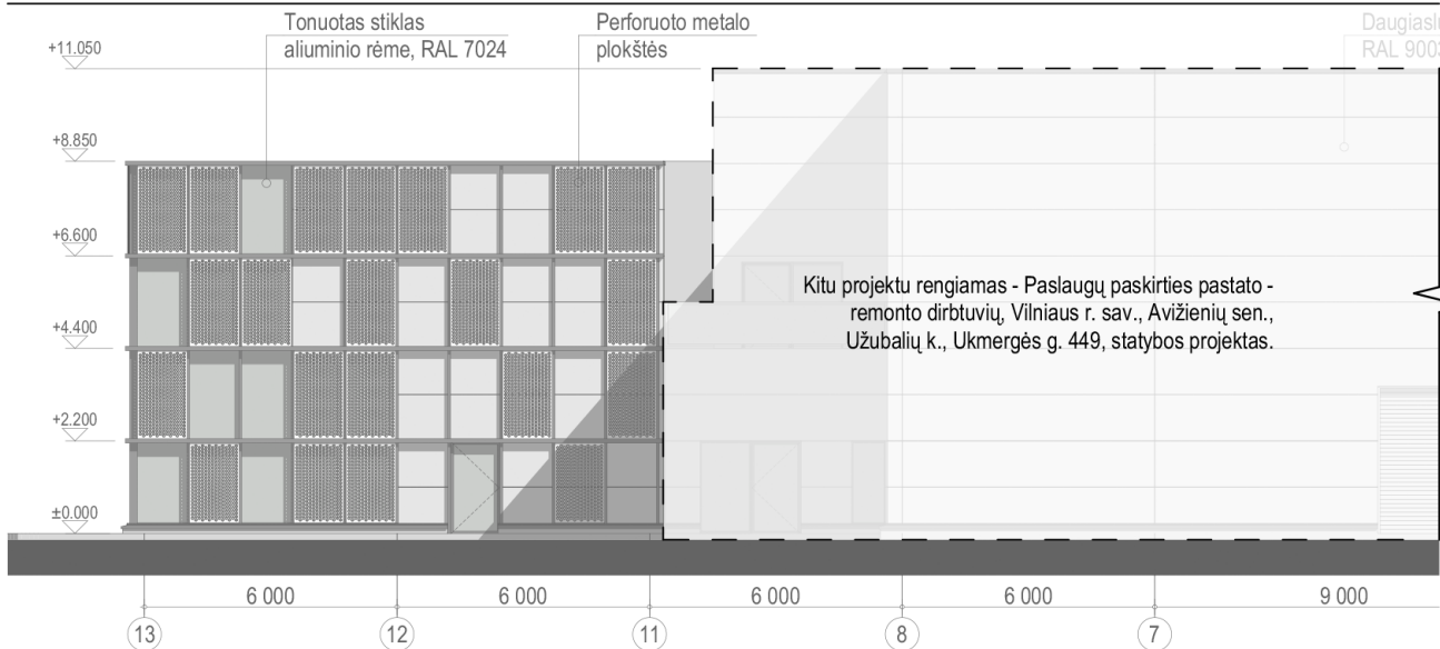
RYTINIS FASADAS
