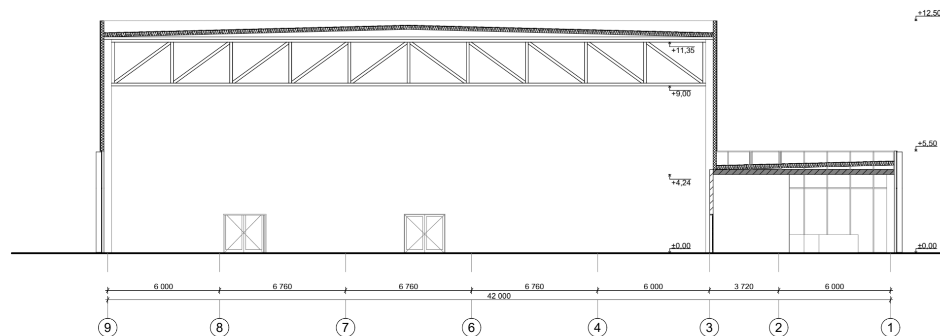
B PJŪVIS 1:200
