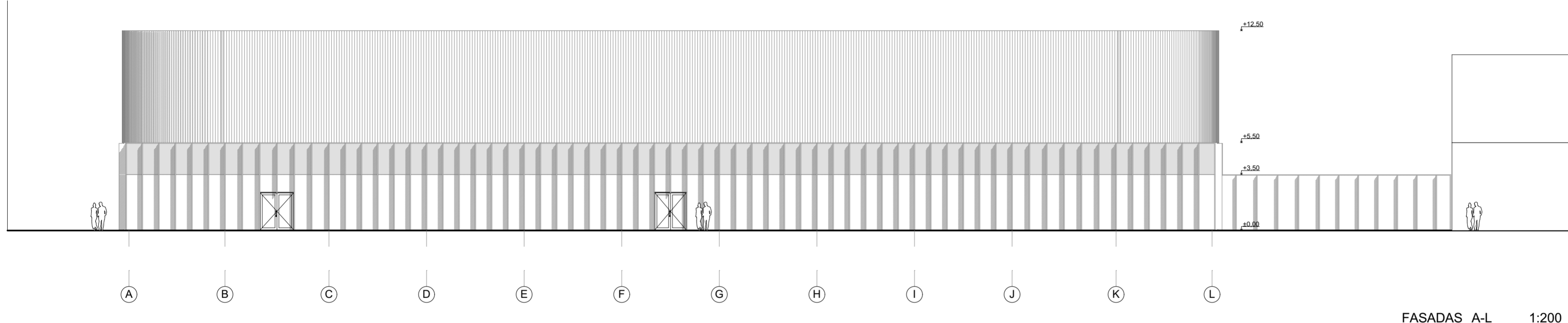
FASADAS A-L 1:200
