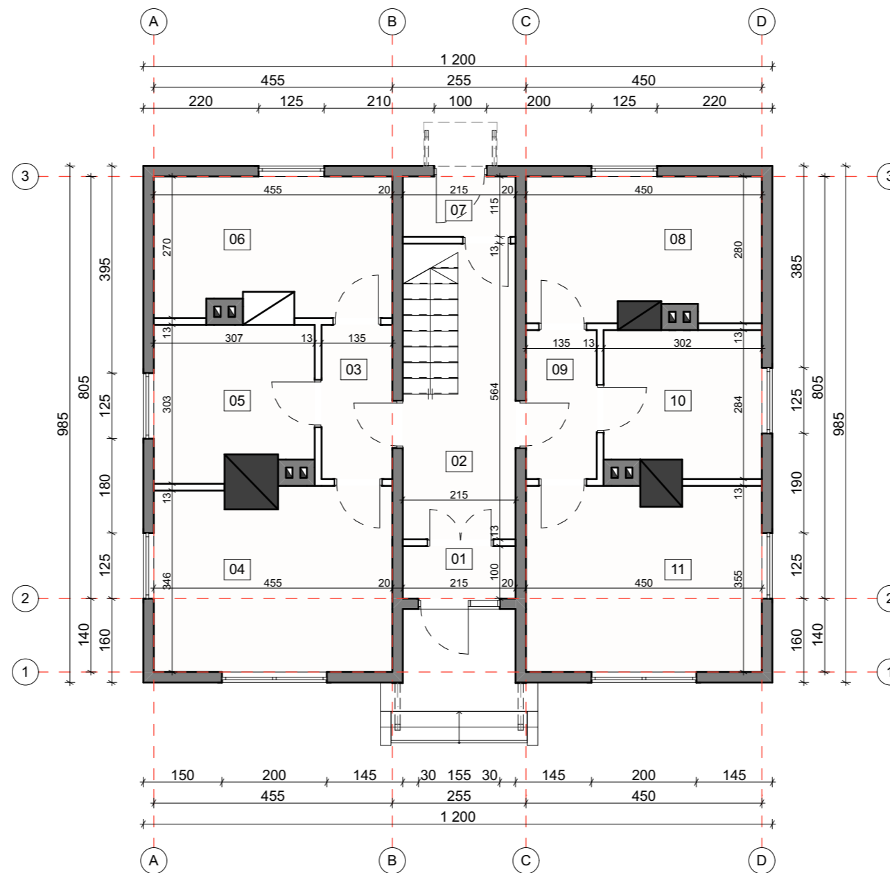
PROJEKTUOJAMAS PIRMO AUKŠTO PLANAS M 1:100
