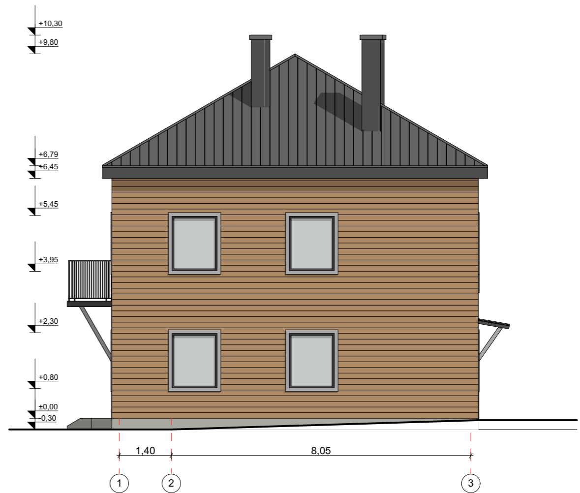
ŠONINIS FASADAS 1-3 M 1:100
