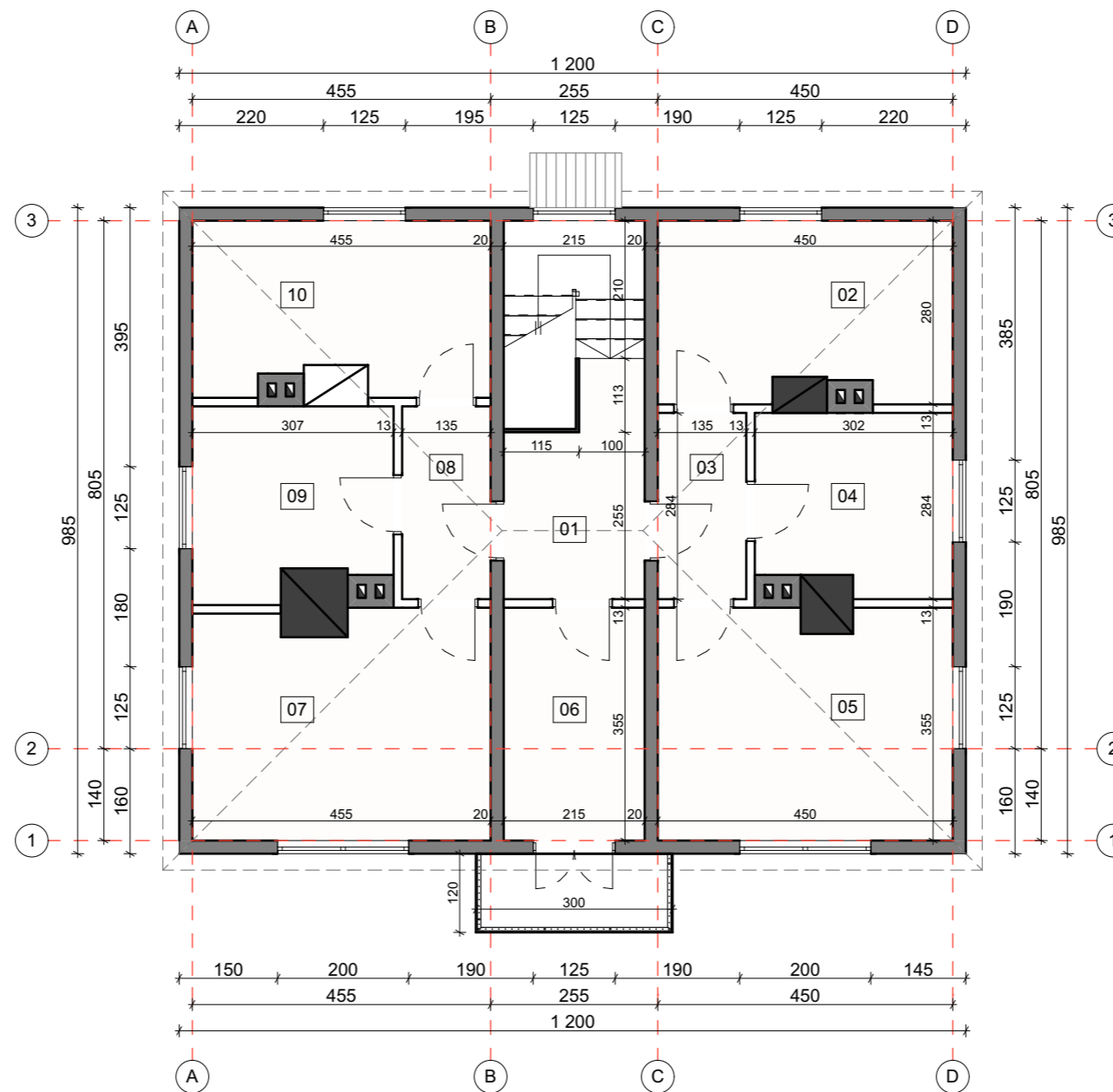
PROJEKTUOJAMAS ANTRO AUKŠTO PLANAS M 1:100
