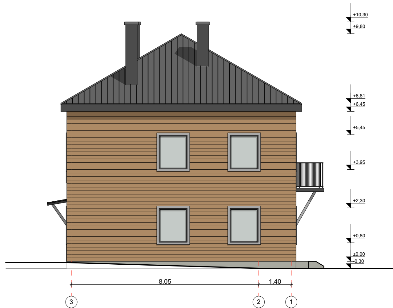
ŠONINIS FASADAS 3-1 M 1:100
