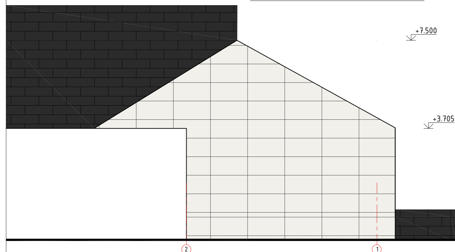
FASADAS 2-1 M 1:100
