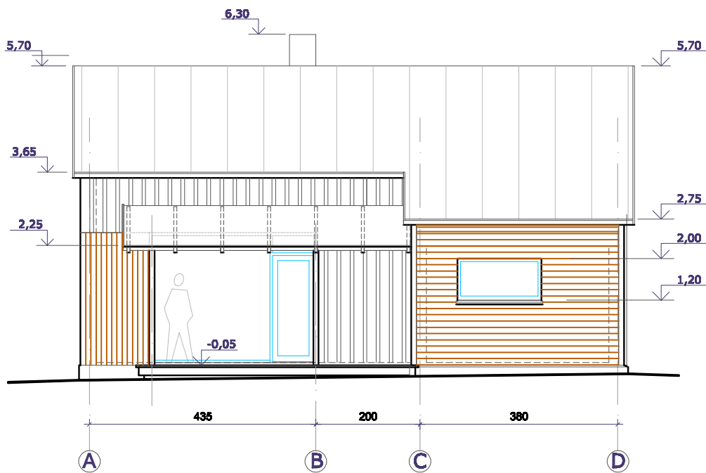
PIETRYČIŲ FASADAS M 1:100
