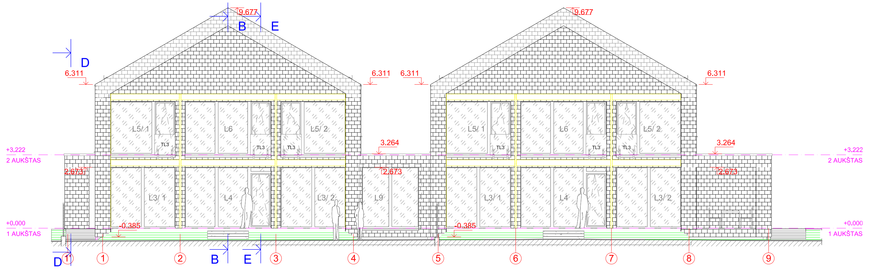
PIETŲ FASADAS AŠYJE A 1 : 100
